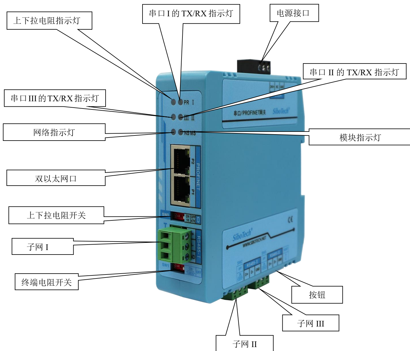
图 1 产品外观
