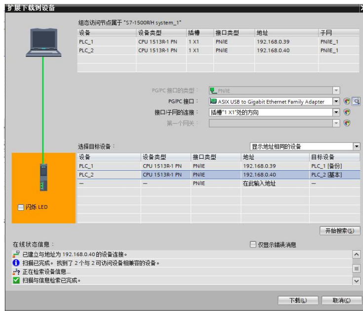
图 20 搜索 PLC
