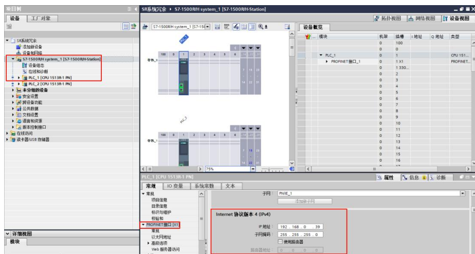
图 6 修改 PLC_1 IP 地址
