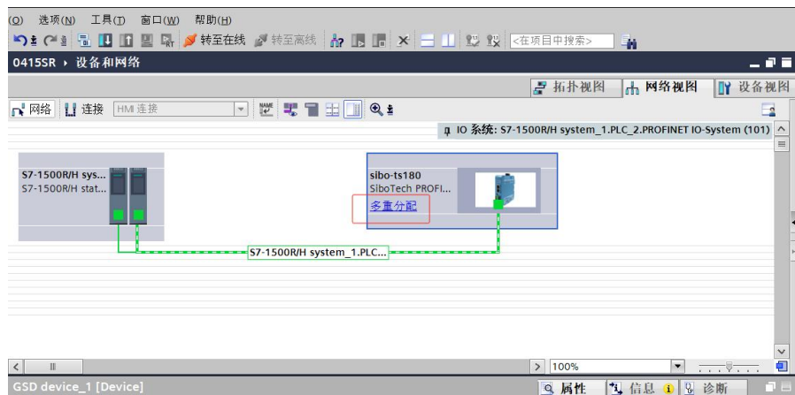
图 12 添加组态
