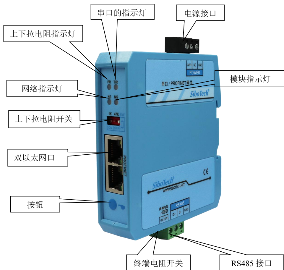
图 1 产品外观
